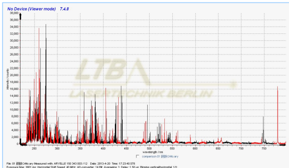
ARYELLE 150 的 LIBS 实测谱图 220nm~800nm
